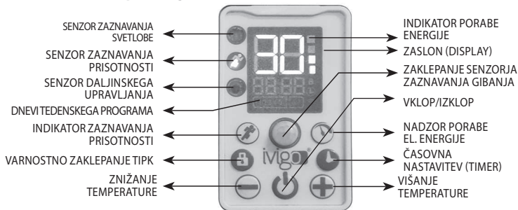
Slika 13: Profesionalna digitalna kontrolna enota
